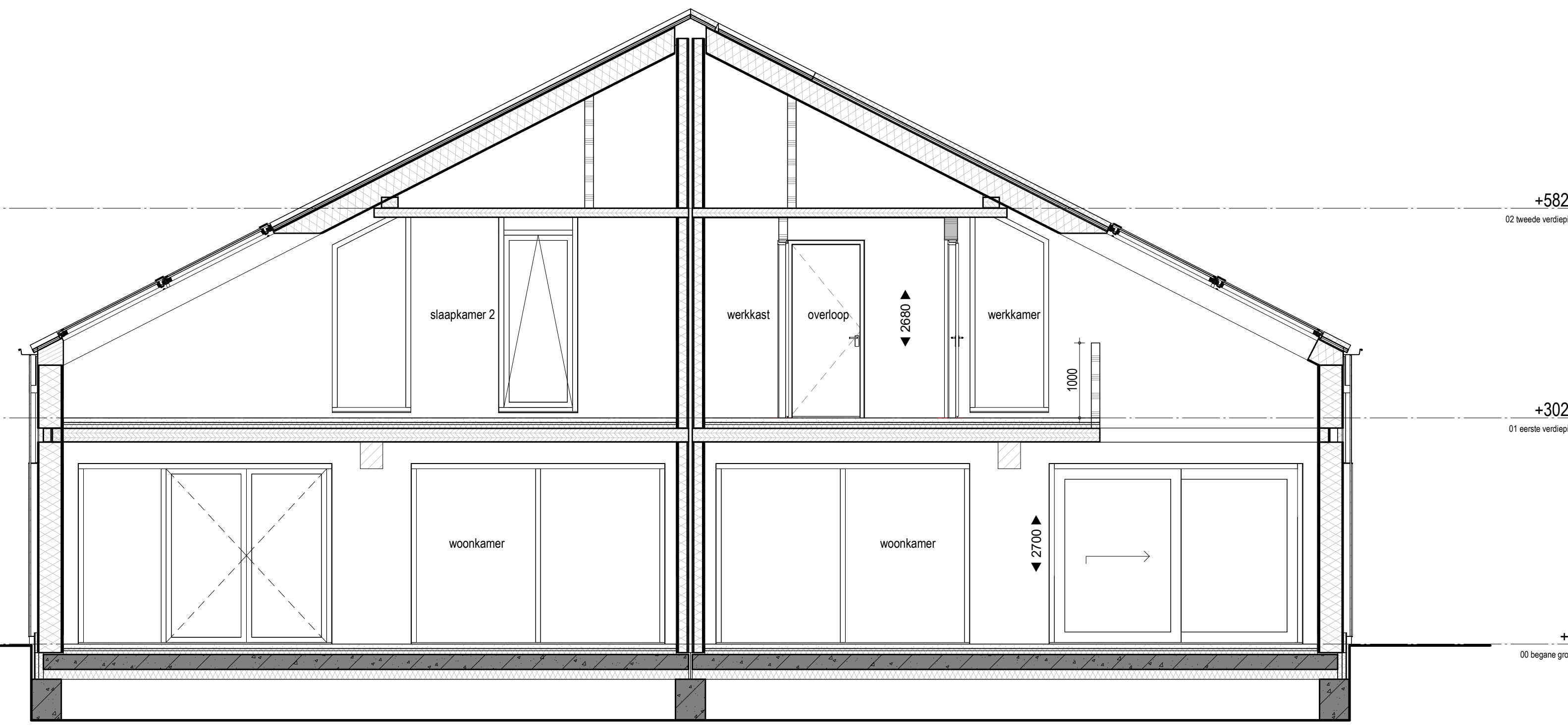
Doorsnede B
