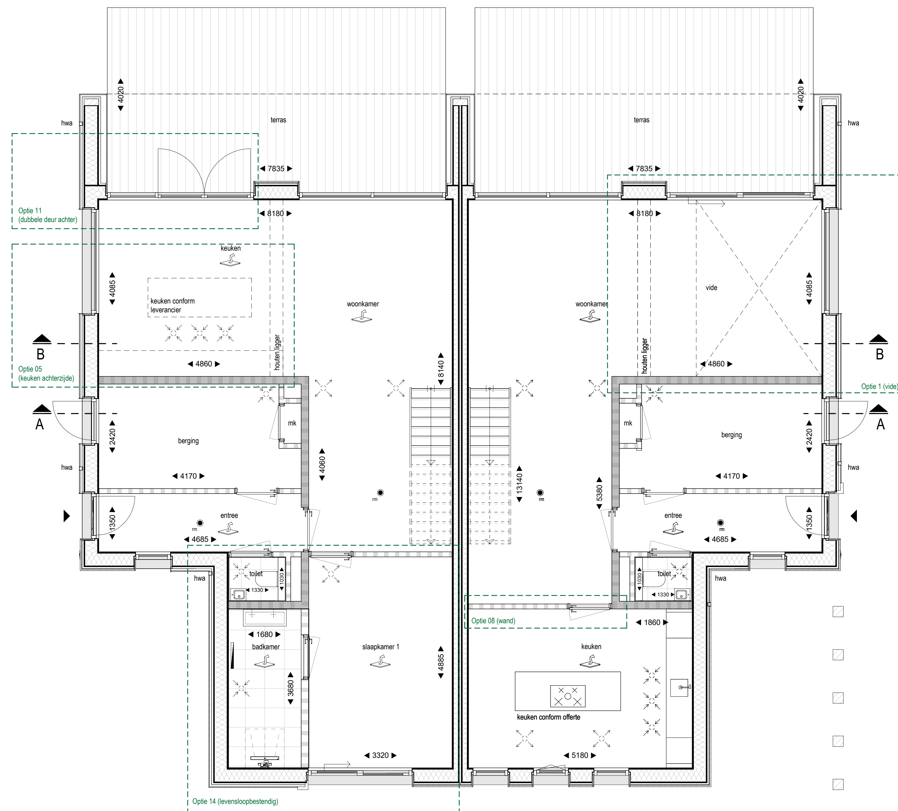
Begane grond
